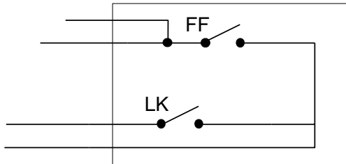
Bild 6. Blockschaltbild mit Linienkontakt (LK) und Fremdfeldkontakt (FF)
