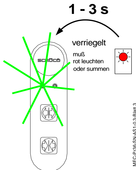
Bild 3. Anwendung kombinierte Öffnungs- und Verschlussüberwachung bei Schüco e-slide Türen.
